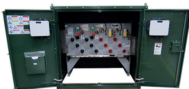
SECCIONADOR TIPO SF6 G&W
